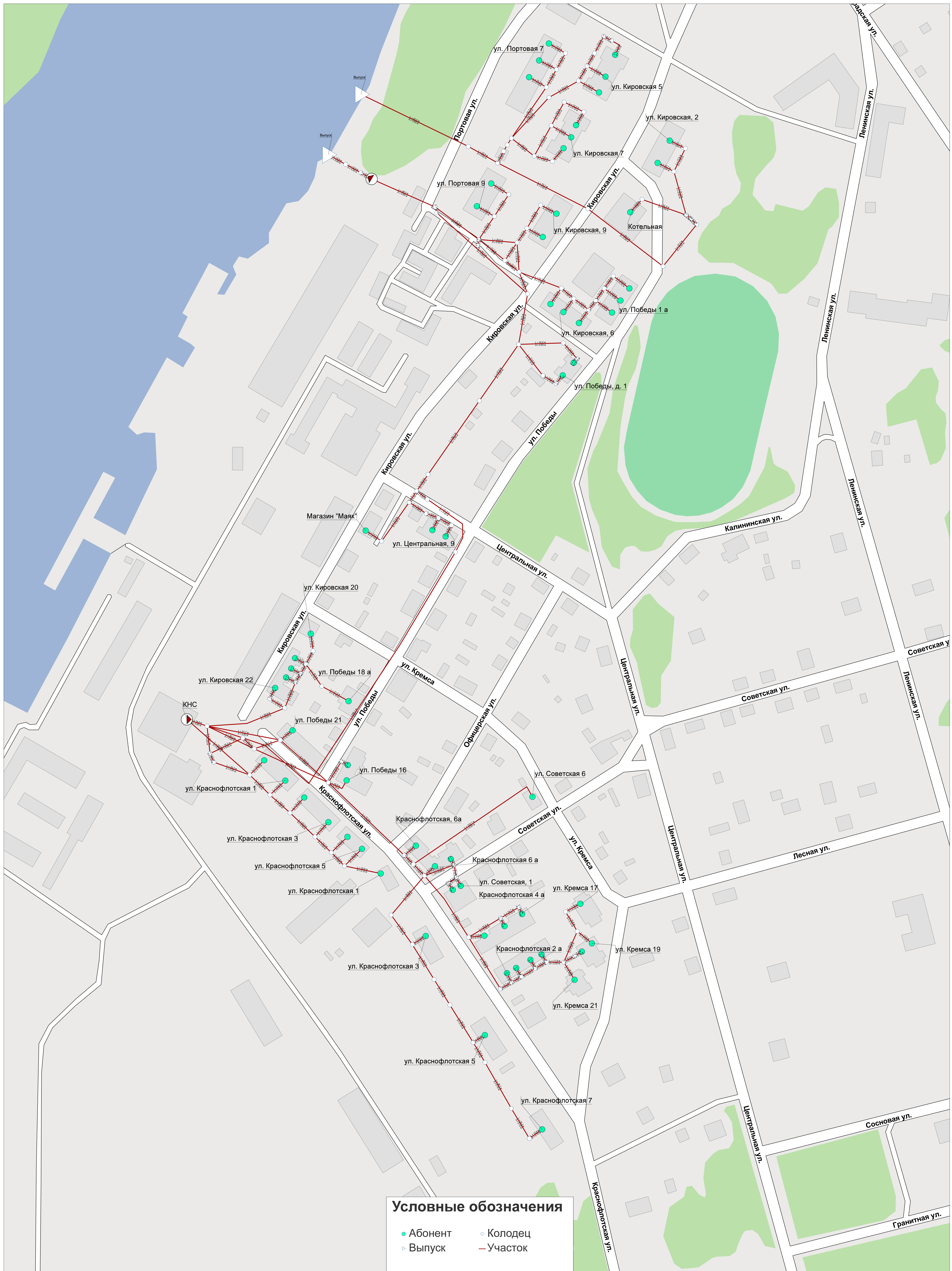
Схема водоотведения г. Высоцк
